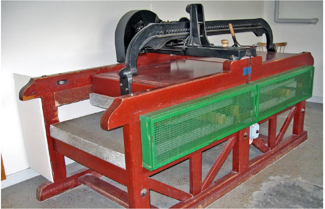
Stenmangeln består av två tunga kalkstenshällar. Mellan dem finns trärullar att placera lakan och annat runt. Nedan till vänster ses manöverpanelen då ena eller andra sidan ska lyftas.
