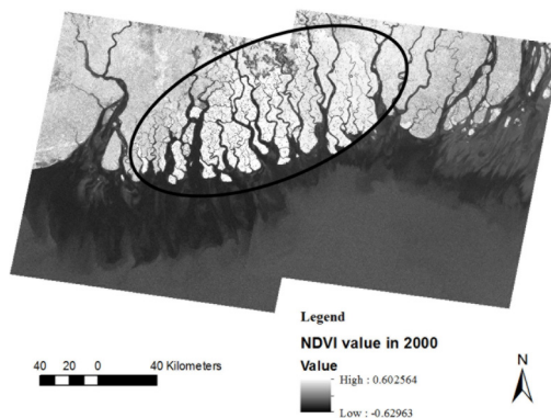
Fig. 3. NDVI values in 2000
